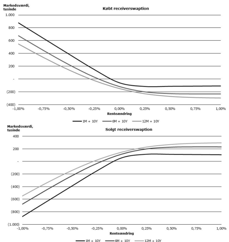
Figur 3. Markedsværdiprofiler ved ændringer i løbetid og markedsrente
